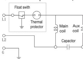
Схема электрической цепи
